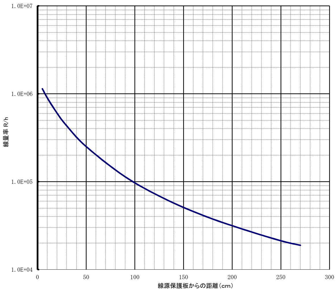
距離－線量率曲線
